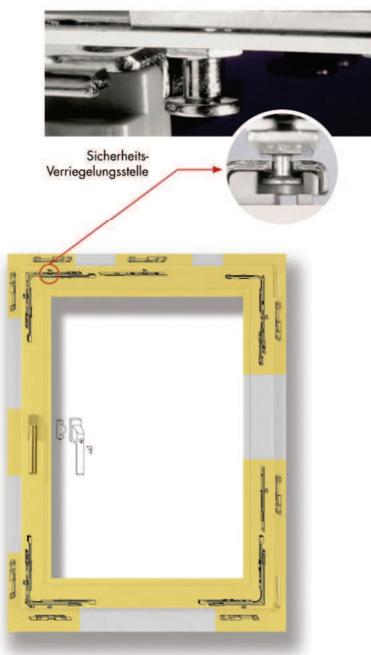
Beispiel eines (Nachrüst-)Fensterbeschlags
